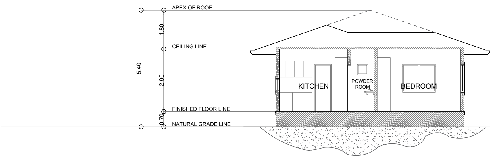
1 CROSS SECTION A3 A4 SCALE 1 : 100 M.
