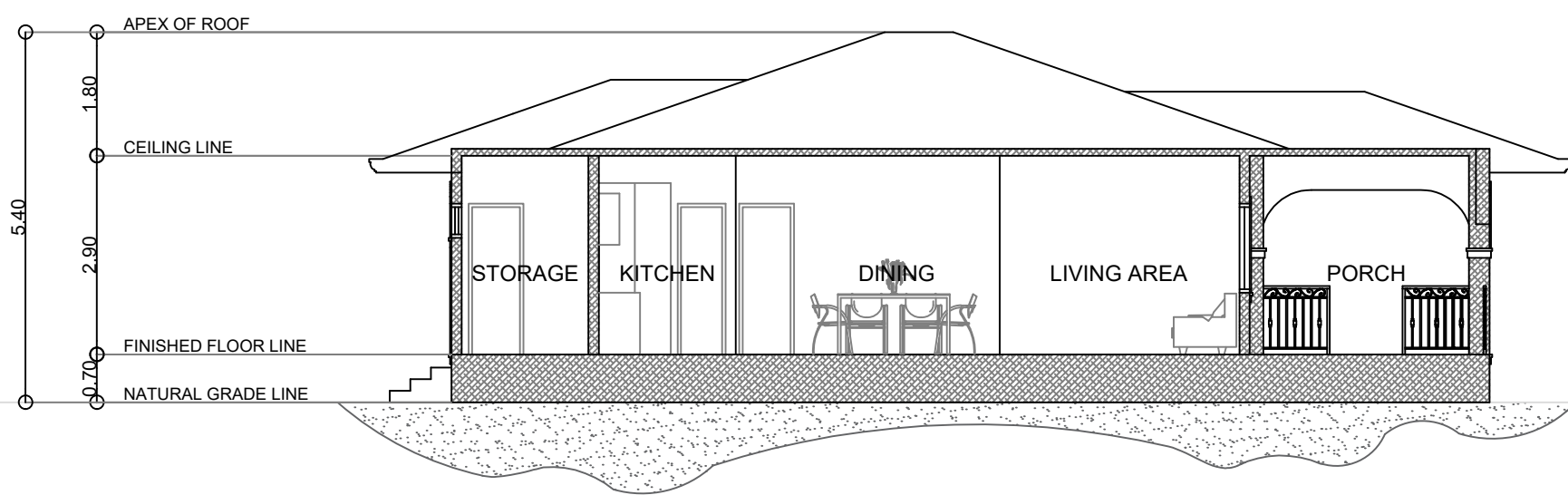
2 LONGITUDINAL SECTION A3 A4 SCALE 1 : 100 M.
